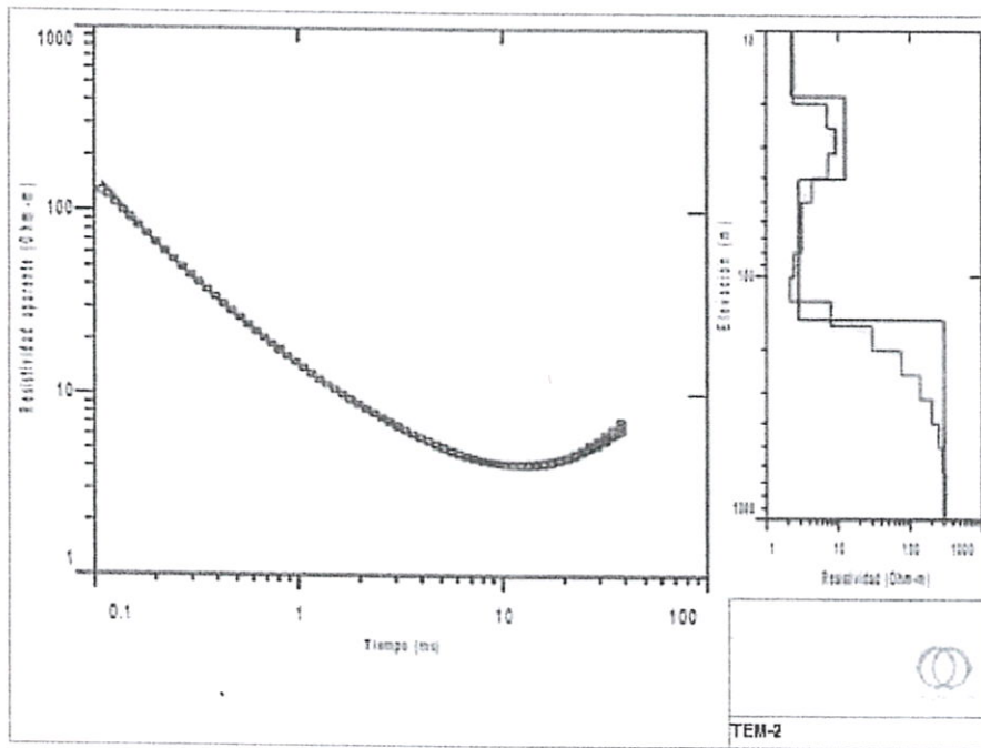
REPRESENTACION GRAFICA DE LOS DATOS OBTENIDOS EN CAMPO EN UNA DIMENSION E INTERPRETACION DE MODELADO DEL PERFIL LITOESTRATIGRAFICO.
