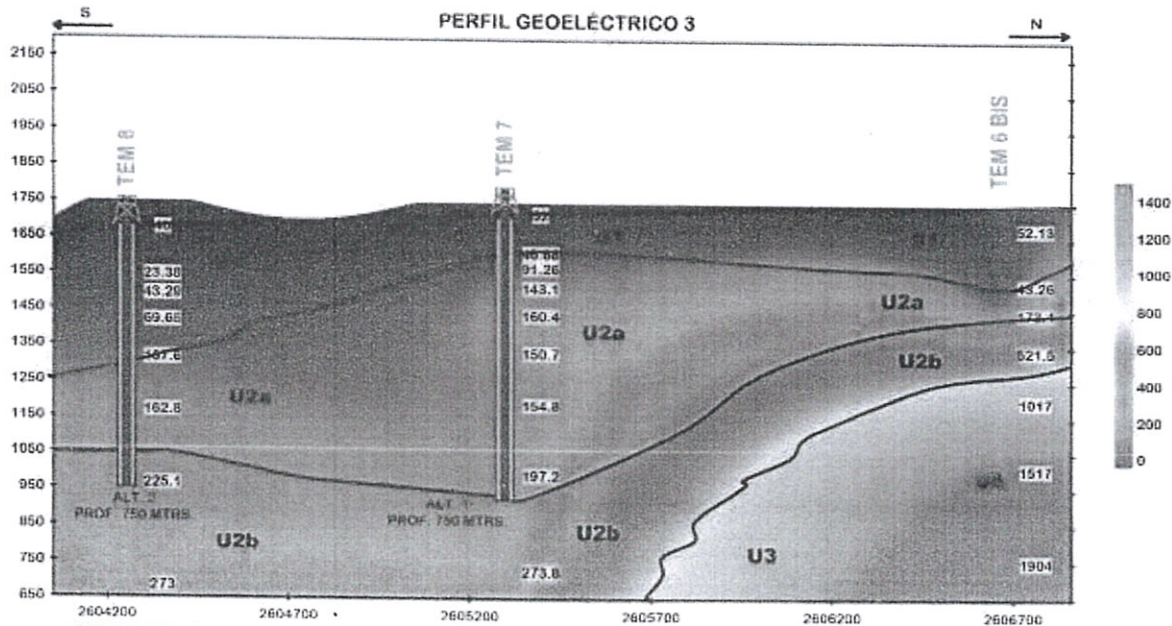
REPRESENTACION GRAFICA DE LA CORRELACION DE INFORMACION EN DOS DIMENSIONES.
